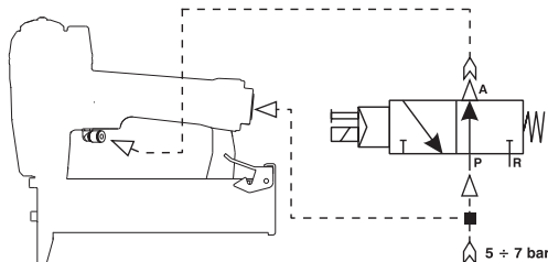
VALVOLA 3/2 NA SZELEP 3/2 NO
