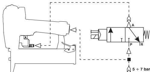
VALVOLA 3/2 NC SZELEP 3/2 NC
